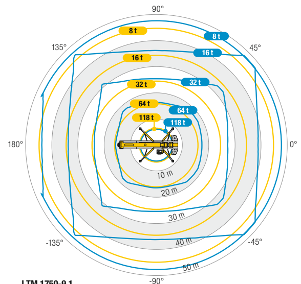
LTM 1750-9.1
